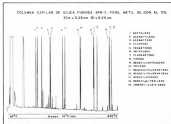
Fig. 2. Cromatograma del estándar de Hidrocarburos Aromáticos Policíclicos
