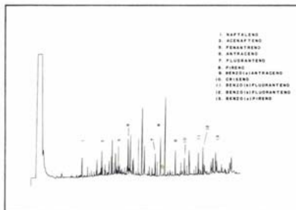
Fig. 3. Cromatograma de HAPs de la estación 12
